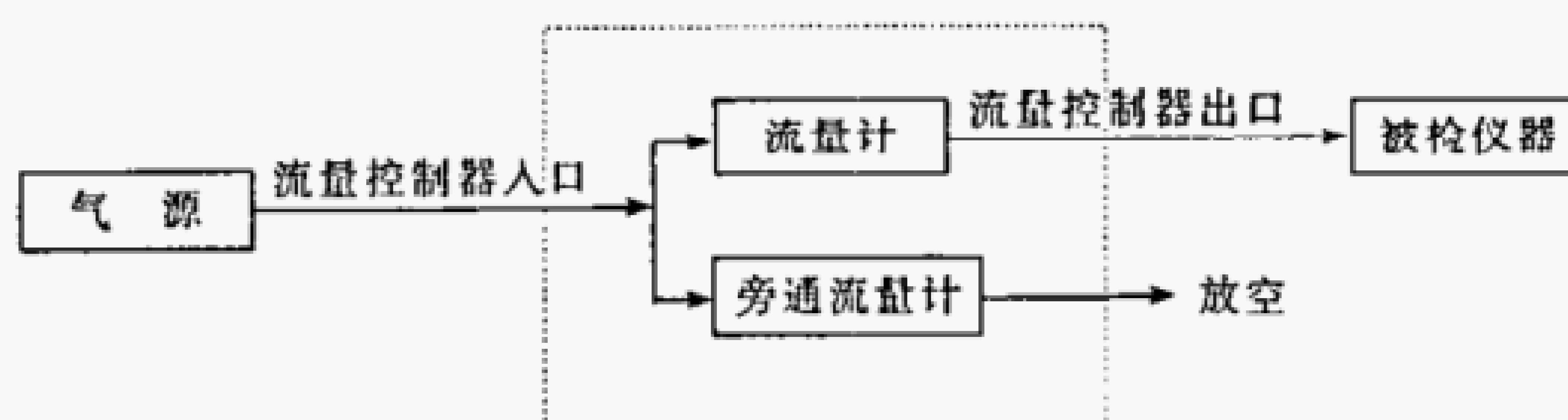
图 A.1 流量控制器
