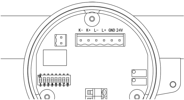
附2： 结构/连接示意图
